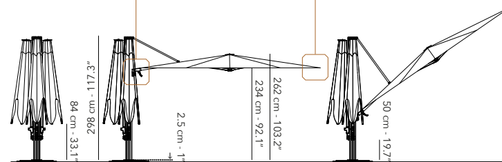
All dimensions exclude the base. - Toutes les dimensions excluent la base. - Alle afmetingen zijn exclusief de parasolvoet.
