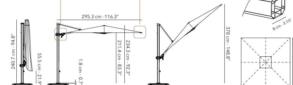
All dimensions exclude the base. - Toutes les dimensions excluent la base. - Alle afmetingen zijn exclusief de parasolvoet.
